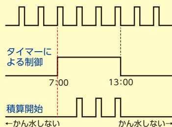
積算日射量による出力
