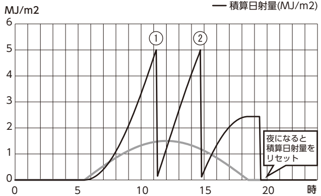
曇りの日のかん水回数
