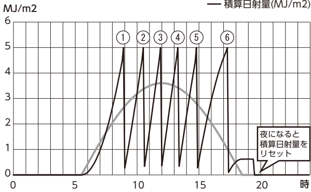
晴れの日のかん水回数
