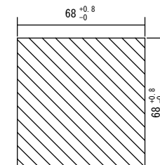
パネルカット寸法 1/2
