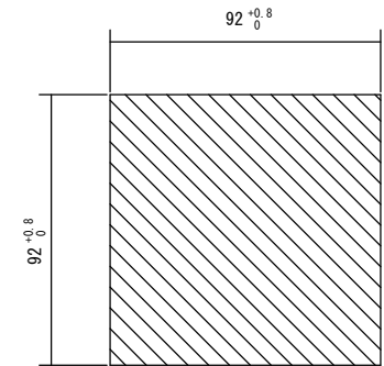
パネルカット寸法 (1/2)
